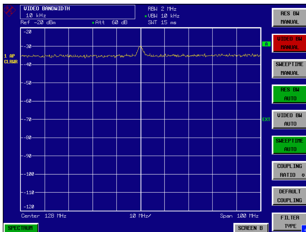
Fig. 2-3 Darstellung eines HF-Sinussignals mit geringem Rauschabstand bei kleiner Videobandbreite.
