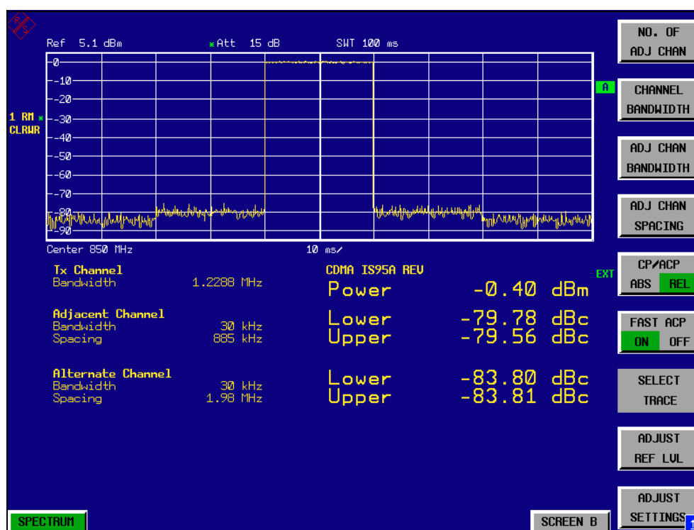
Fig. 2-8 Messung der Kanalleistung und des Nachbarkanalleistungsabstandes bei IS95-Signalen im Zeitbereich (Fast ACP)
