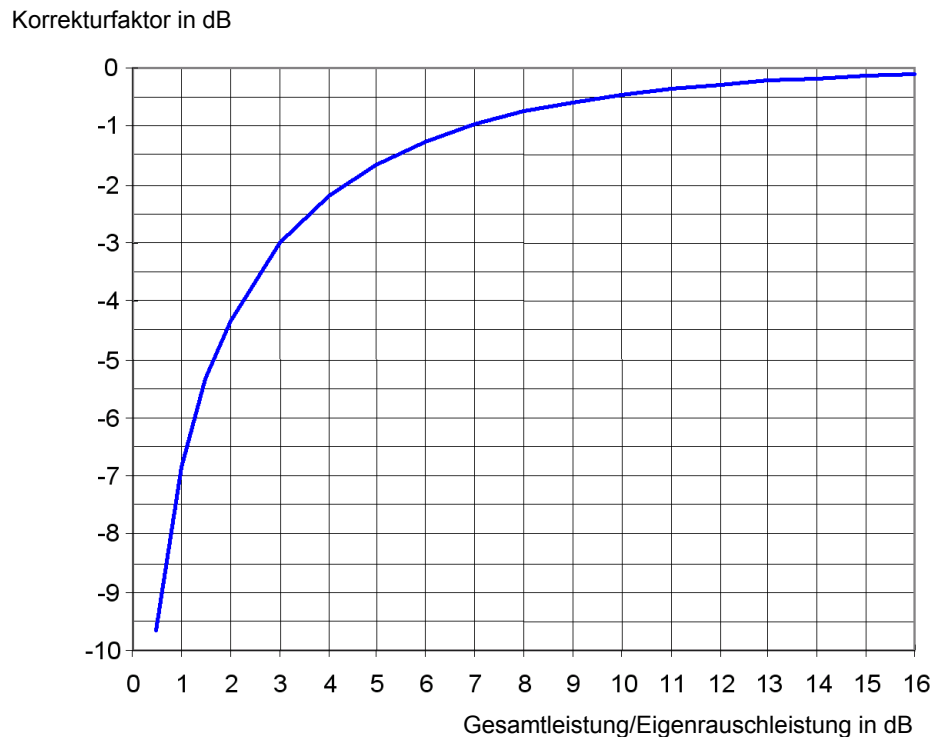
Fig. 2.15 Korrekturfaktor für die gemessene Rauschleistung abhängig von Abstand zu Eigenrauschleistung des R&S FSQ
