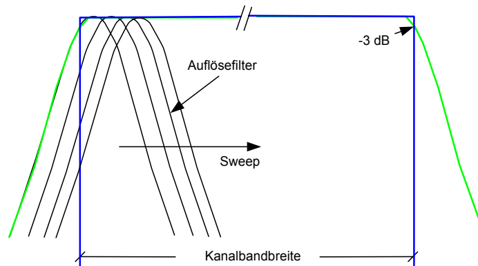
Fig. 2.16 Approximation des Kanalfilters durch Sweeplen mit kleiner Auflösesebandbreite
