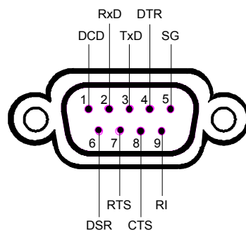
Bild 8.7 Pinbelegung der RS-232-Schnittstelle
