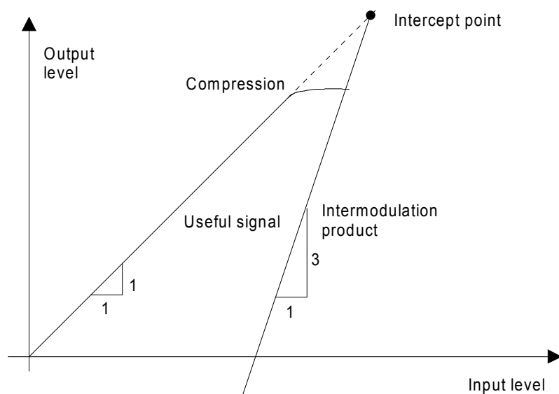
Bild 4.17 Abhängigkeit des Pegels der Störprodukte vom Pegel der Nutzsingale
