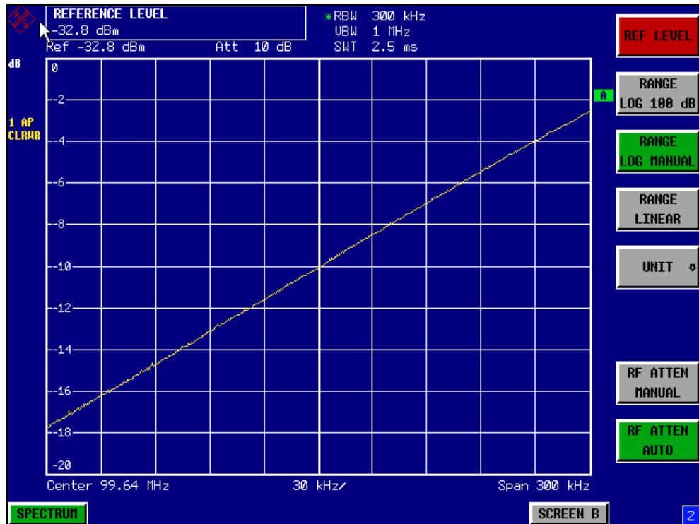
Fig. 2-4 Darstellung der Filterflanke des 300\text{-kHz} -Filters als FM-Diskriminatorkennlinie.
